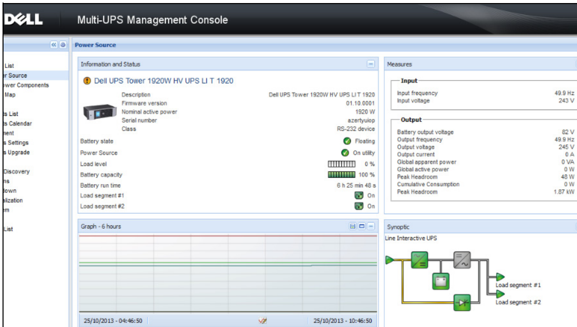
図 18. 電源の表示
